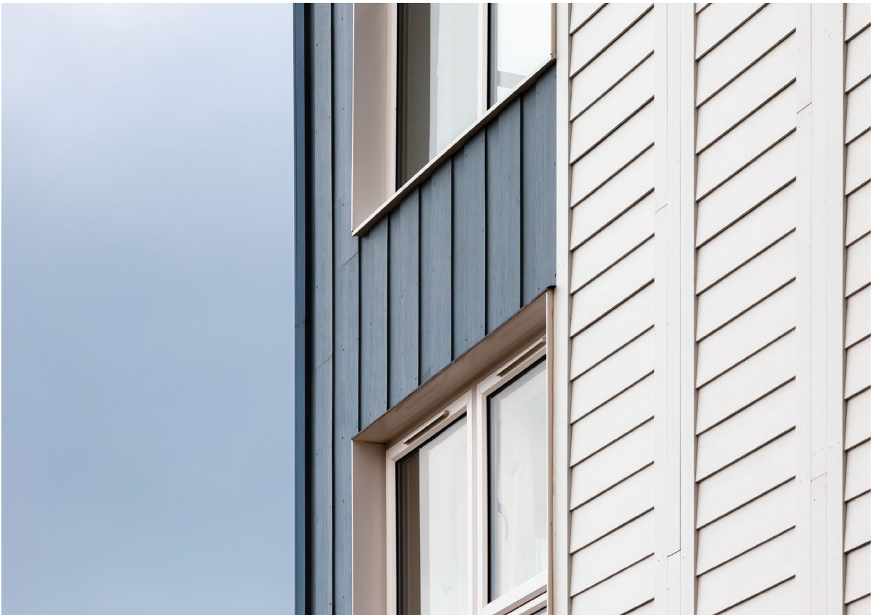
Hardie® Plank Fassadenplatten als Kombination von Boden-Deckel-Schalung und Stülpschalung
